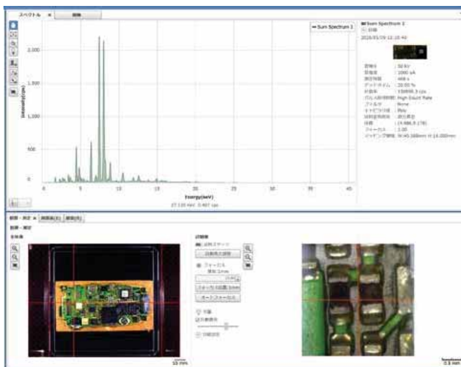
図4：測定画面
