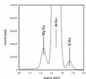
図2：Mgピーク付近スペクトル (アルミニウム合金、Mg4.9%含有)
