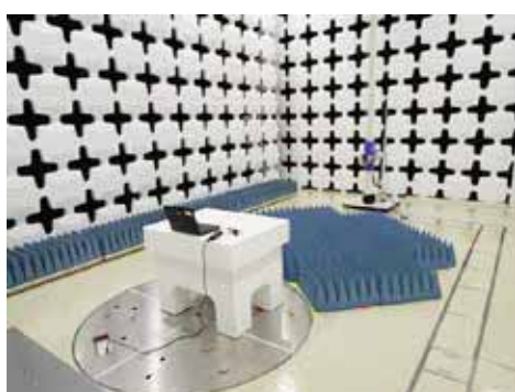
図1：1GHz超の放射妨害波測定(3m法電波暗室)
