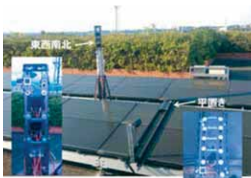
図1：海老名本部屋上におけるPSCモジュール屋外暴露試験の様子
