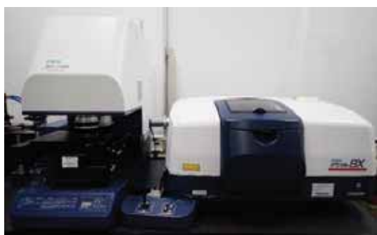
図1：フーリエ変換赤外分光分析システム(日本分光(株)製) 右側：FT/IR-8X(マクロ測定用) 透過、ATR、拡散反射、RAS測定が可能 左側：IRT-7100(赤外顕微鏡) 透過、反射、ATR測定が可能
