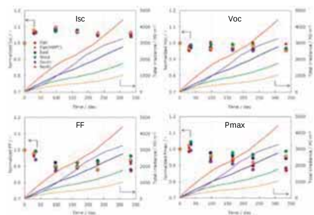
図4：標準試験条件におけるPSCモジュールの規格化短絡電流(Isc)、開放電圧(Voc)、曲線因子(FF)、最大出力(Pmax)の経時変化と積算日射量の比較
