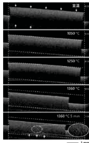
図2: 急速昇温条件で加熱したイットリア安定化ジルコニア成形体の内部構造と外形の変化
