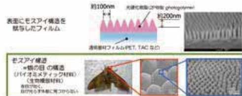
図2：モスアイ型反射防止フィルムの構造
