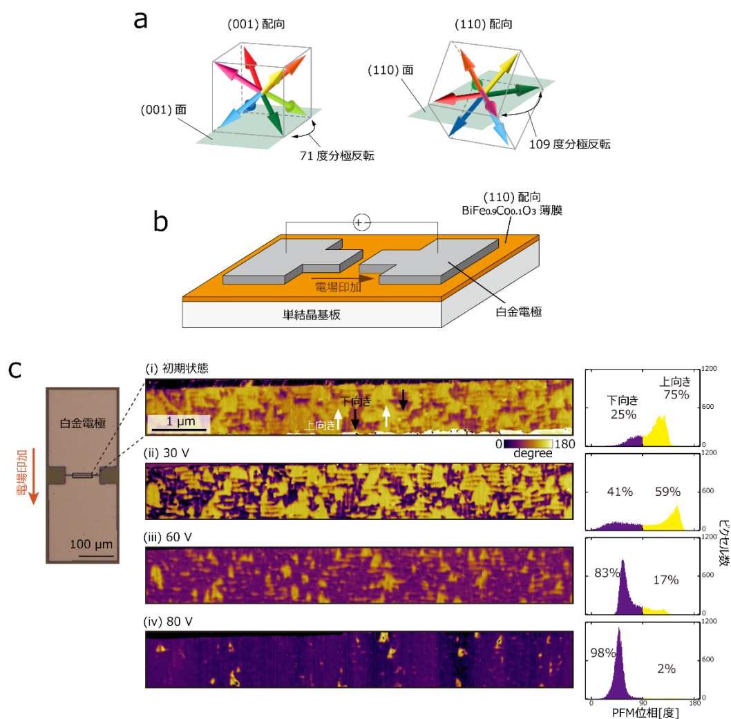
図 1. (a) \text{BiFe}_{0.9}\text{Co}_{0.1}\text{O}_3 の(001)配向と(110)配向の違い。立方体は結晶構造の最小単位を、8 色の矢印は電気分極の取りうる向きを表す。(b) 109 度分極反転のための白金電極の配置。(c) 実際の白金電極の顕微鏡写真と、電場印加による強誘電ドメインの分布の変化(圧電応答顕微鏡図)。黄色と紫色はそれぞれ上向き・下向きの分極を表しており、右図にはその分布のヒストグラムを示している。
