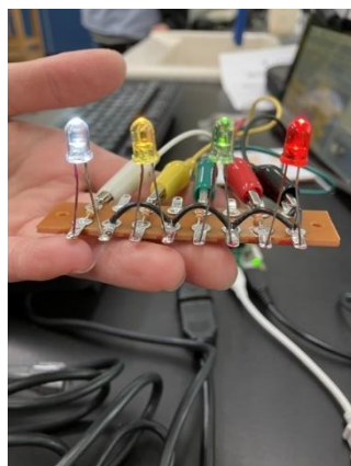
・LED 点灯回路
